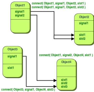
Obrázek: Signály a sloty v Qt
